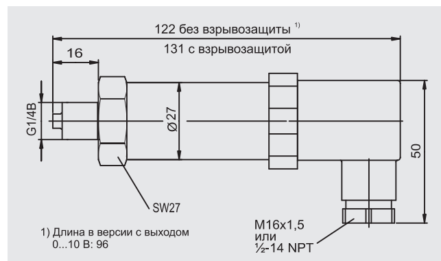
Измерительный преобразователь 7MF1564-... с подключением к процессу G1/4" (внешняя), размеры в мм
